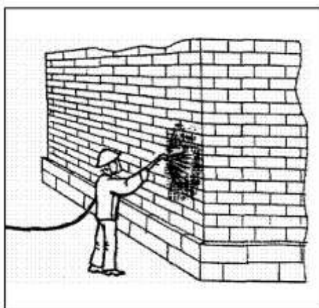
Рис. 12. Технологическая схема гидрофобизации кирпичной стены
